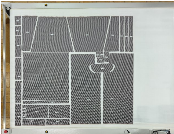
「ふたばのかぜ」のパターンは、直線で構成されハグレのない設計に。曲線の余り部分は胸ポケットに。
